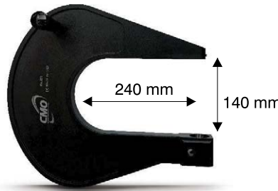
◀ Trancia 10 Ton idraulica per il taglio della lamiera. Utilizzabile per la foratura con punzoni da 0,6 mm e da 0,8 mm. Questo accessorio è necessario per la foratura della nuova lamiera in alluminio e per la calibratura dei fori esistenti delle lamiere in alluminio e in acciaio. Foratura della lamiera in acciaio al boron fino a 3 mm.
